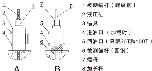
图2-11 连接图解
